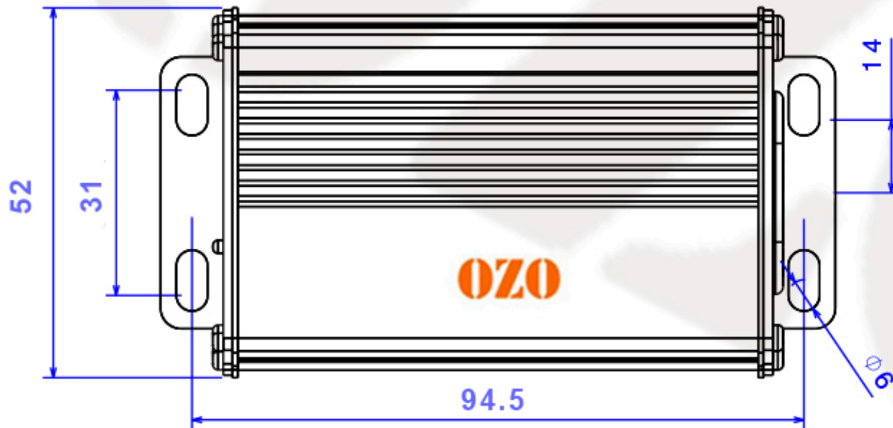
Vue de dessus Echelle : 1:1
