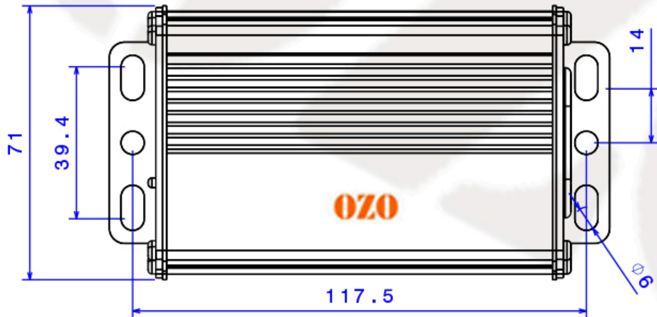
Vue de dessus Echelle : 1:1
