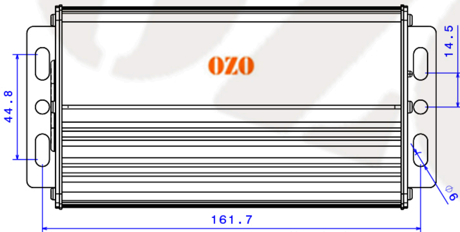
Vue de dessus Echelle : 1:1
