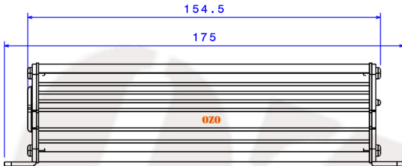
Vue de profil Echelle : 1:1
