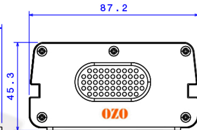
Vue de face Echelle : 1:1
