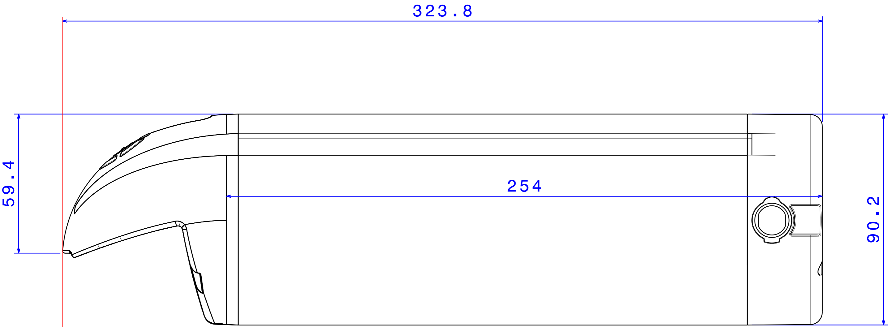
Vue de profil Echelle : 1:1
